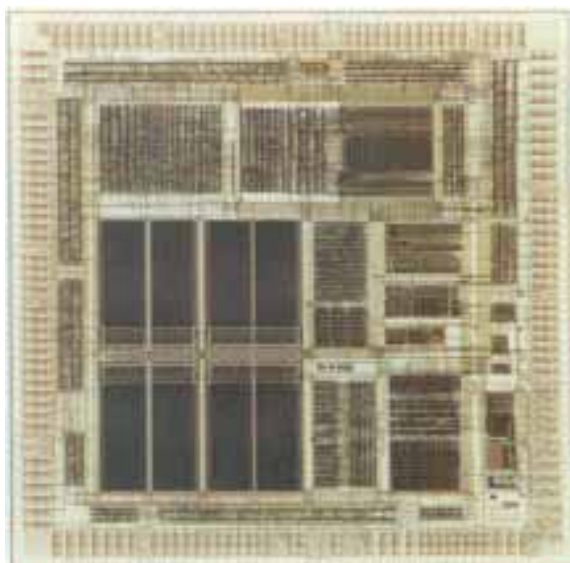
図 2. SH マイコン第一号(SH1)
